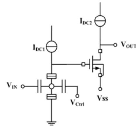
parallel SETMOS
