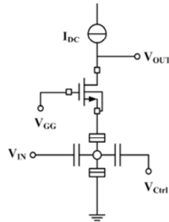
serial SETMOS
